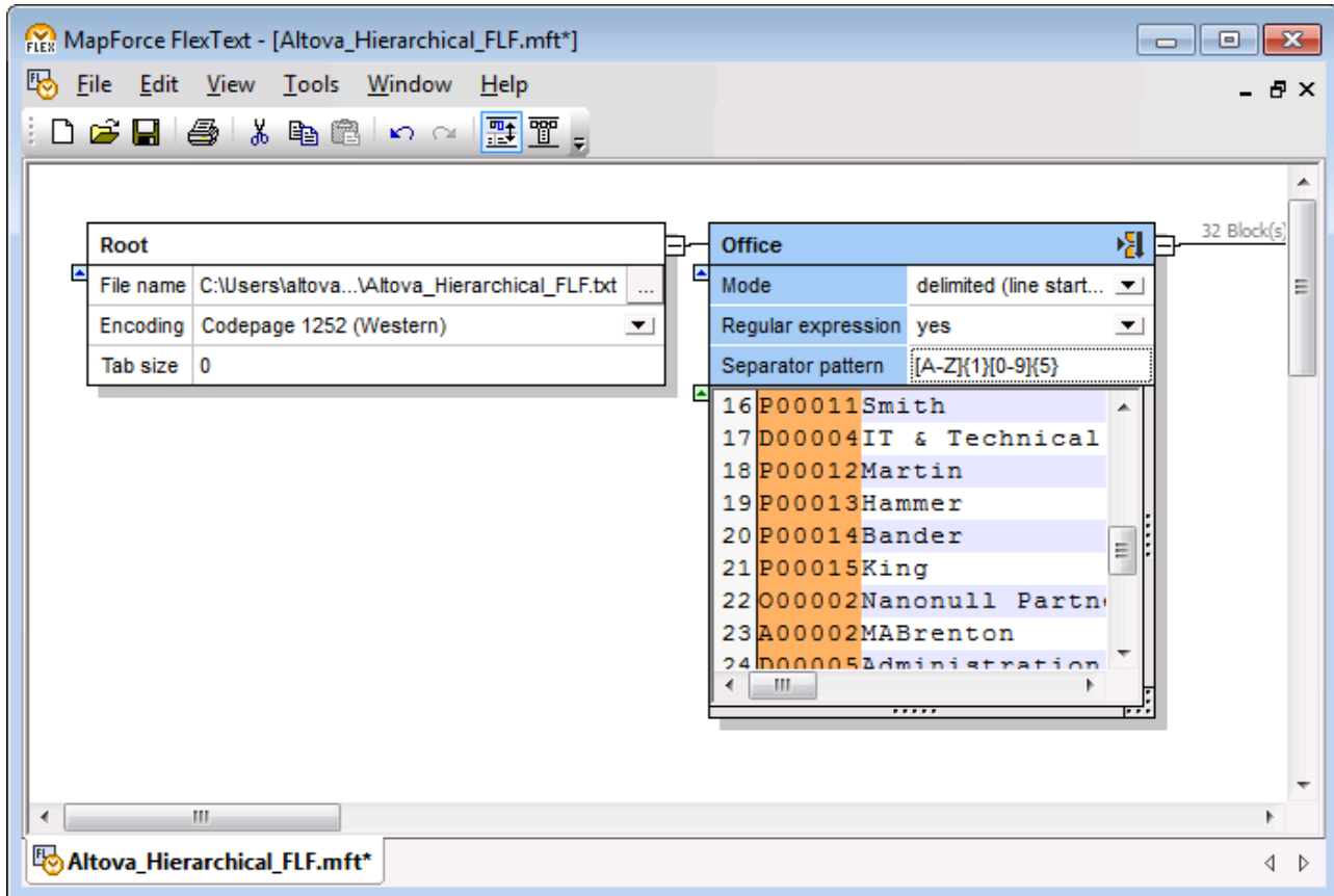
Modèle d'échantillon FlexText qui utilise des expressions régulières pour séparer du texte
