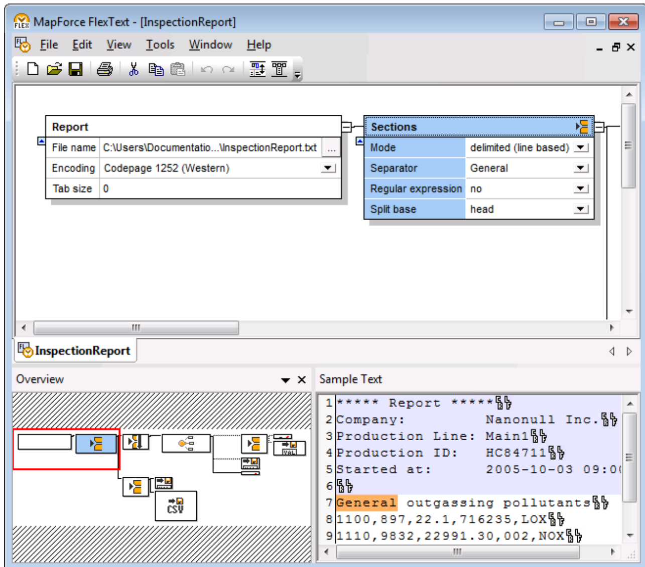
L'interface graphique FlexText
