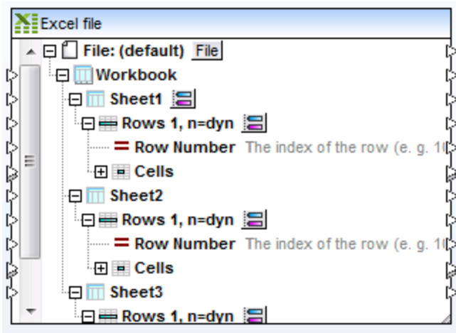
Composant Excel par défaut
