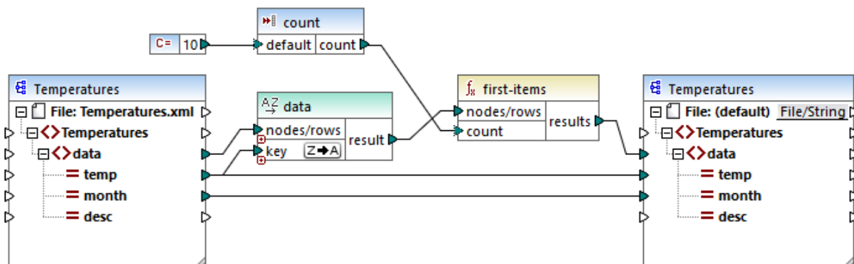
FindHighestTemperatures.mfd
