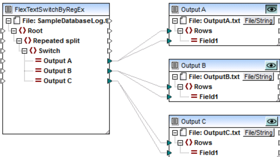
FlexTextSwitchByRegEx.mfd
