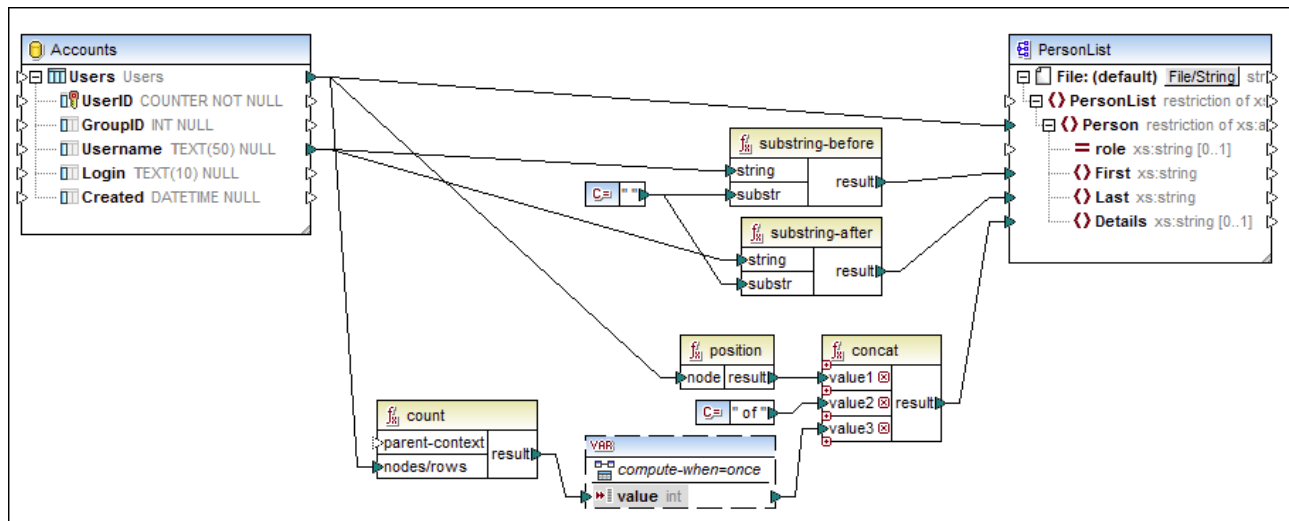
DB_UserList.mfd
