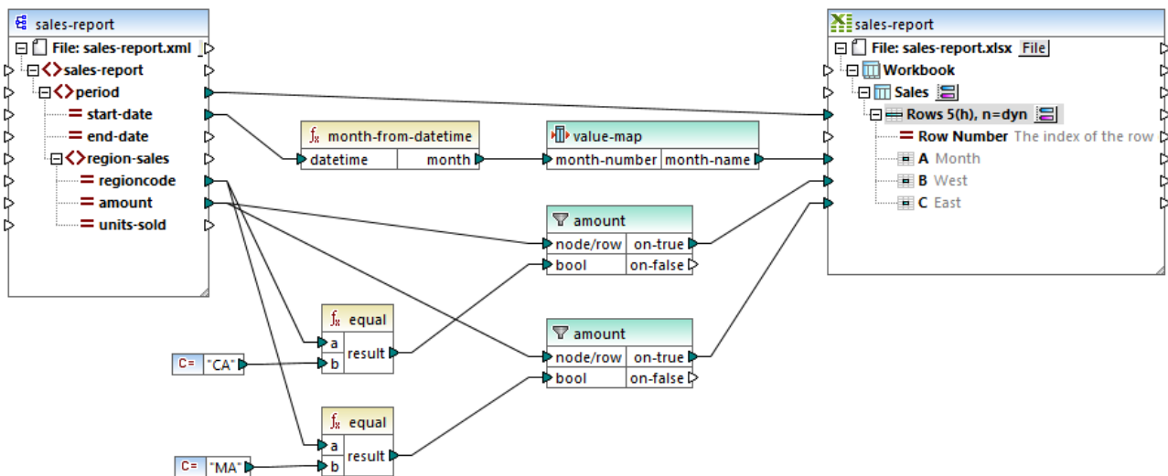
Sales_to_Excel.mfd
